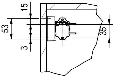
E ( 1 : 5 )
