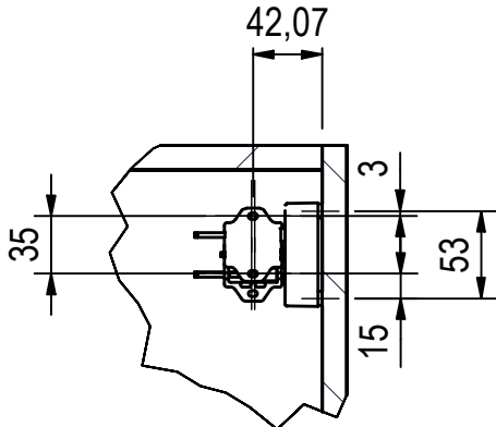
D ( 1 : 5 )
