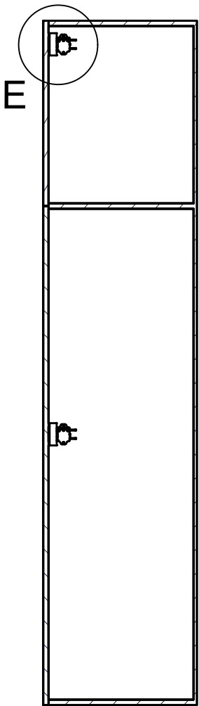
B-B ( 1 : 15 )
